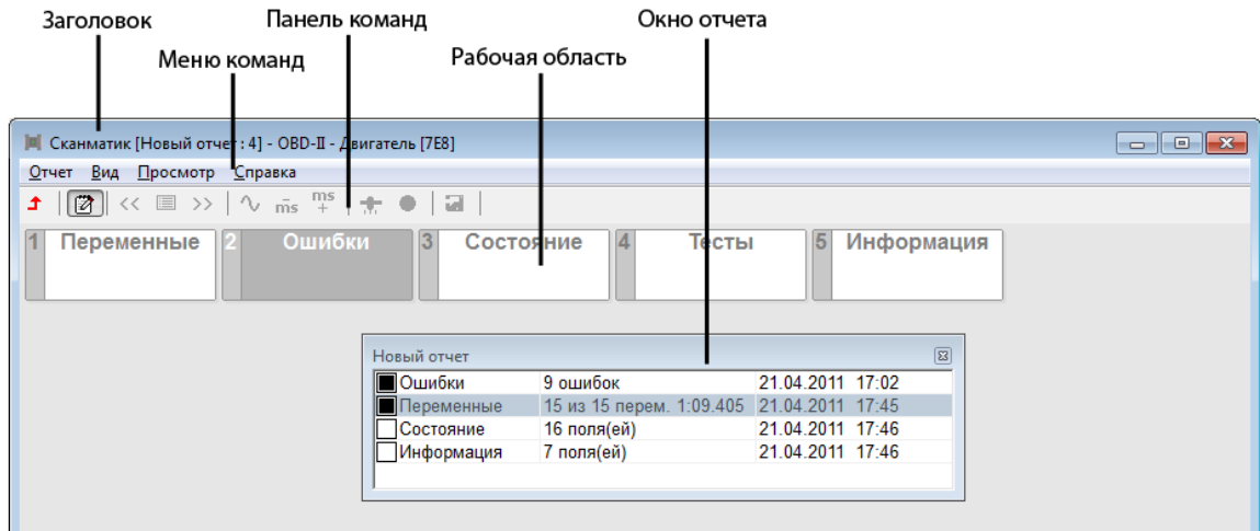
Интерфейс программы
